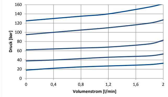
Druckstufe 120 bar
