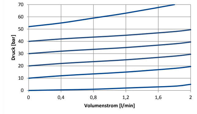
Druckstufe 70 bar
