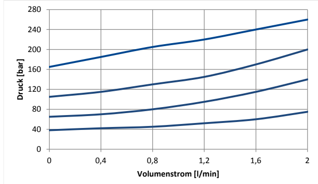
Druckstufe 200 bar
