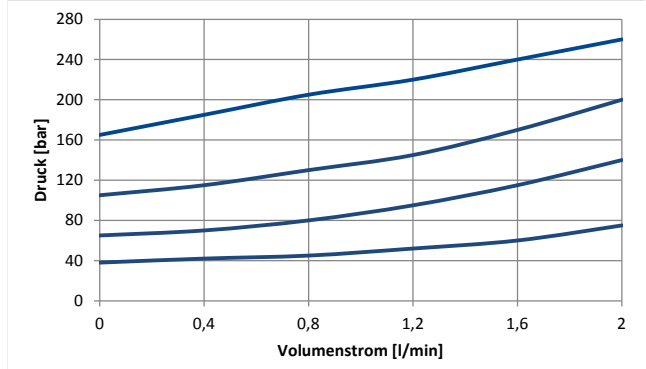
Druckstufe 200 bar
