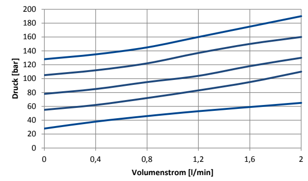
Druckstufe 150 bar
